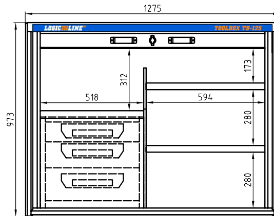
ToolBox TB-125 Fachsystem V2 (Art.Nr. 01 043 12 00)
