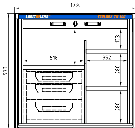
ToolBox TB-100 Fachsystem V2 (Art.Nr. 01 044 12 00)
